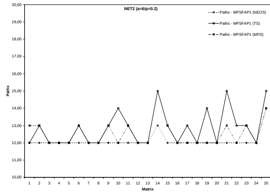
(d) Paths, a = 6
