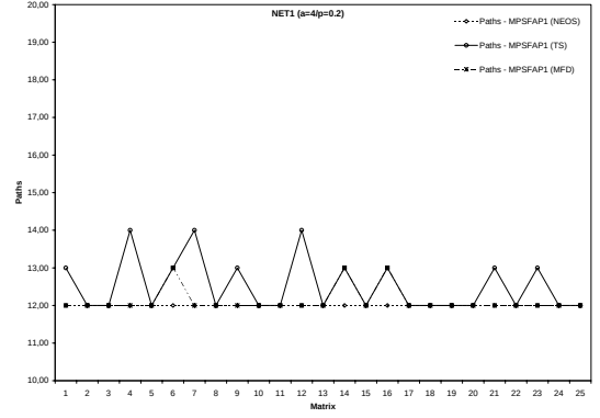
(d) Paths, a = 4
