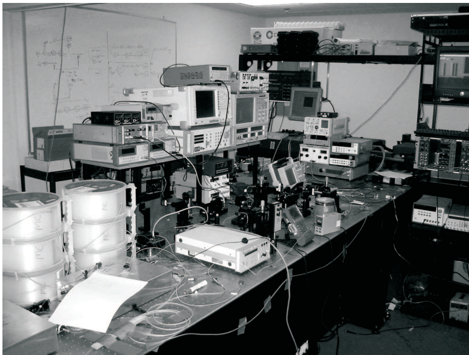
FIG. 8.8 – Photo de l'expérience réalisée sur une distance de 76 km de fibre optique (on voit les rouleaux de 3 bobines de 25 km, l'un des rouleaux étant utilisé pour envoyer le signal de synchronisation).
