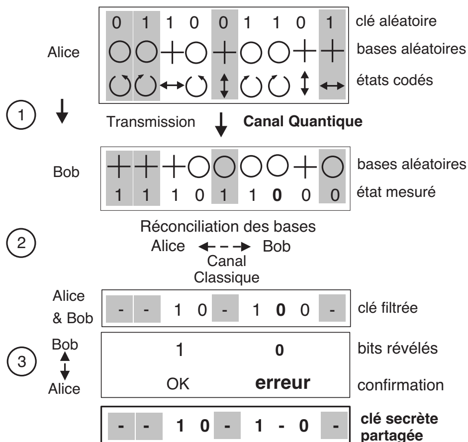
FIG. 6.2 – Résumé des différentes étapes du protocole BB84 conduisant au partage d'une clé secrète entre Alice et Bob.
