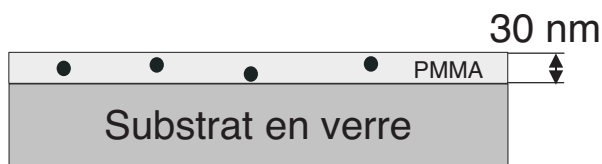
FIG. 3.4 – Échantillons réalisés pour l'observation de molécules uniques, obtenus par dépôt sur une lamelle de verre d'une solution de colorant dilué dans du PMMA
