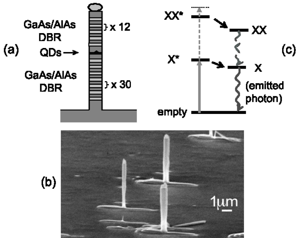
FIG. 2.6 – Emission de photon uniques dans les boîtes quantiques InAs en micropiliers. (a) Diagramme schématique de la structure d’une boîte quantique unique dans un micropilier et principe de fonctionnement de la source de photons uniques par un processus de cascade radiative. (b) Image des micropiliers enregistrée par microscopie électronique à balayage. Les micropiliers ont une hauteur d’environ 5\ \mu\text{m} et un diamètre qui peut varier de 0.3 à quelques microns. Ces figures sont extraites de la référence [112].
