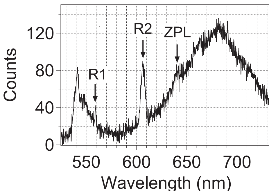
FIG. 5.2 – Spectre de fluorescence d’un centre NV unique dans un nanocristal de diamant. Le centre coloré est excité en éclairage continu à la longueur d’onde \lambda = 514.5 nm et à une puissance d’excitation de 10 mW. Ce spectre a été obtenu à l’aide du spectrographe imageur + matrice CCD représenté sur la figure 3.5. On devine la raie à zéro phonon (ZPL) et plus nettement les raies de diffusion Raman à un phonon R1 et à deux phonons R2 provenant de la matrice cristalline de diamant. Le pic étroit qui apparaît en dessous de 550 nm provient de lumière parasite du laser d’excitation, à 514.5 nm, diffusée dans le spectrographe.
