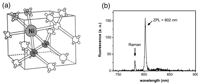
FIG. 9.1 – (a) Centre coloré NE8 dans la maille cristalline du diamant. Le centre NE8 est un complexe associant un atome de nickel et 4 atomes d'azote voisins. (b) Spectre de fluorescence du centre NE8 excité par un laser continu à la longueur d'onde de 710 nm. Ces figures sont extraites de la référence [93].
