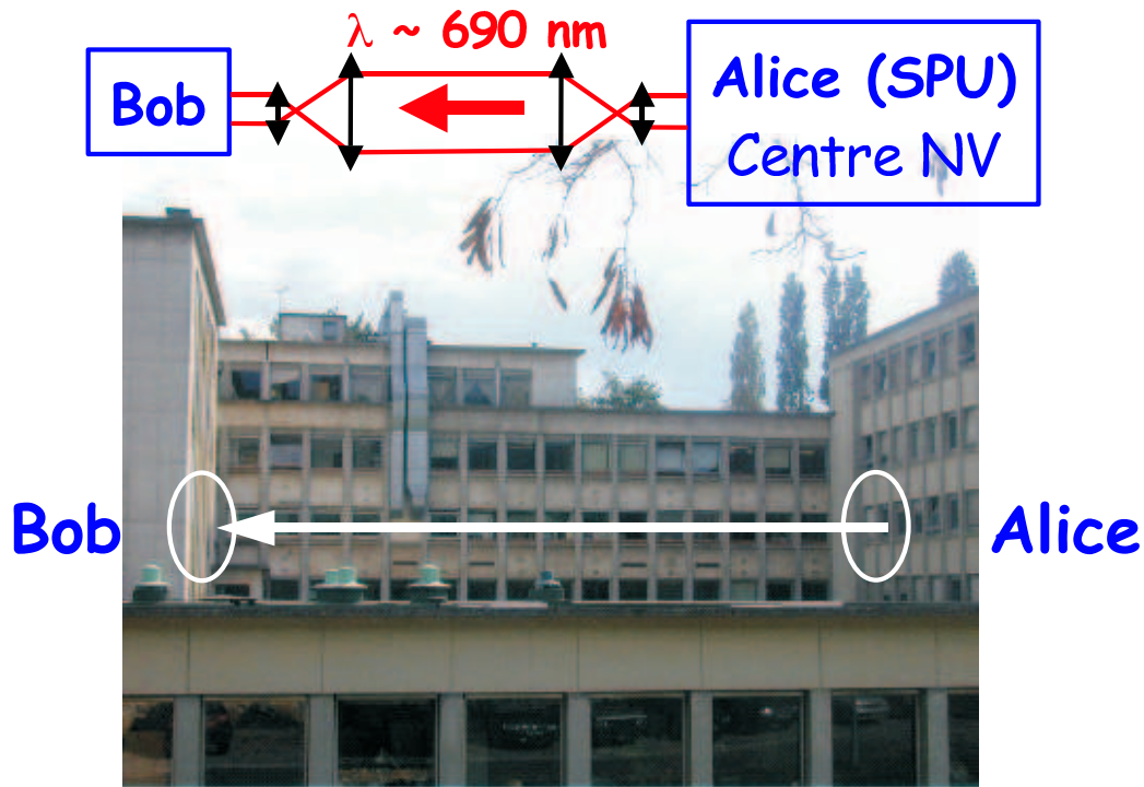
FIG. 7.1 – Disposition relative d’Alice et Bob à l’Institut d’Optique, dans l’expérience, réalisée en octobre 2003, de distribution quantique de clé de cryptage en espace libre. Les deux protagonistes sont séparés par une distance de 30 m.
