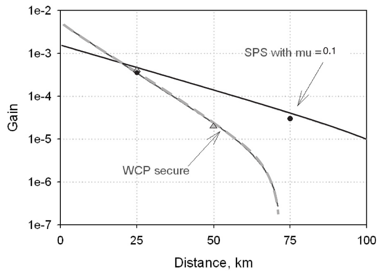
FIG. 8.9 – Comparaison des performances du dispositif décrit dans la figure 8.5.3 en fonction de la distance de propagation, dans le cadre du modèle de sécurité décrit dans la référence [185]. La courbe noire en trait plein représente la performance de la source de photons uniques (SPS) dont le nombre moyen équivalent de photons par impulsion est de 0.1 (voir texte). La courbe grisée, en pointillé, représente les performances accessibles à l'aide d'impulsions cohérentes atténuées. Ces courbes théoriques sont calculées à partir des mesures expérimentales correspondant aux points placés sur la figure : triangles gris pour les impulsions cohérentes atténuées et cercles noirs pour les mesures réalisées à partir de la source de photons annoncés.
