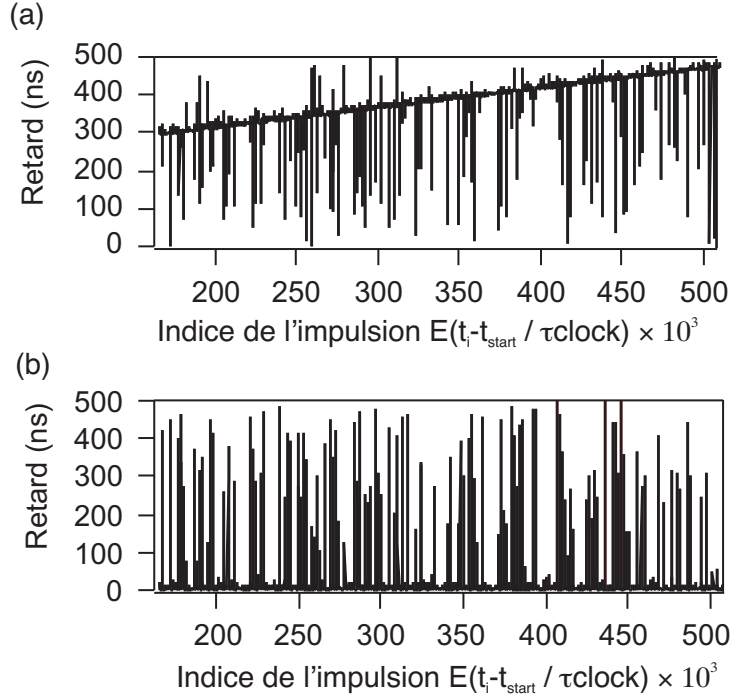
FIG. A.1 – Procédure de synchronisation des instants de photodétection \{t_i\} : on s'intéresse à la valeur du retard \text{Delay}(t_i) en fonction de l'indice de l'impulsion excitatrice E[(t_i - t_{\text{start}})/\tau_{\text{clock}}] pour un couple de paramètres t_{\text{start}} et \tau_{\text{clock}} . (a) Cas où \tau_{\text{clock}} est proche de \tau_{\text{rep}} , ce qui entraîne une petite dérive linéaire de la valeur du retard. En revanche la valeur de t_{\text{start}} est incorrecte. (b) Cas où \tau_{\text{clock}} = \tau_{\text{rep}} avec un précision relative atteignant 10^{-9} et où t_{\text{start}} est correctement évalué.
