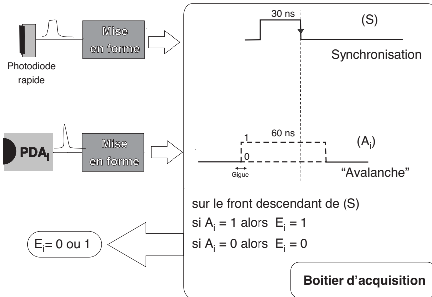
FIG. 7.5 – Schéma détaillant le principe de la mise en forme des signaux de photodétection obtenus chez Bob. Le signal de synchronisation (S) est fourni par une photodiode rapide détectant les impulsions nanosecondes prélevées sur le faisceau d’excitation et envoyées par Alice. Ces impulsions correspondent ainsi à une horloge à 5.3 MHz, cadence d’excitation de la source de photons uniques. Le signal (A i ) de chacune des quatre photodiodes à avalanche (PDA i ) placées chez Bob est transformé en une impulsion TTL de durée égale à 60 ns. Le boîtier d’acquisition permet de régler le décalage temporel relatif de ces deux signaux et d’assurer ainsi une détection « fenêtrée » des clics des photodiodes à avalanche. Chacune des sorties du boîtier d’acquisition fournit les signaux E i pour i = 1, \dots, 4 , lesquels sont ensuite envoyés à une carte d’acquisition « TIA » à quatre voies d’entrées, placée dans un micro-ordinateur (cf. figure 7.2).
