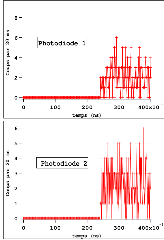
FIG. 3.8 – Autocorrélation avec lui-même du signal de photodétection d'une photodiode à avalanche en régime d'excitation continu. L'absence de coïncidences pour un temps inférieure à 240 ns est la signature d'un temps mort de nature électronique, causé par le TIA.
