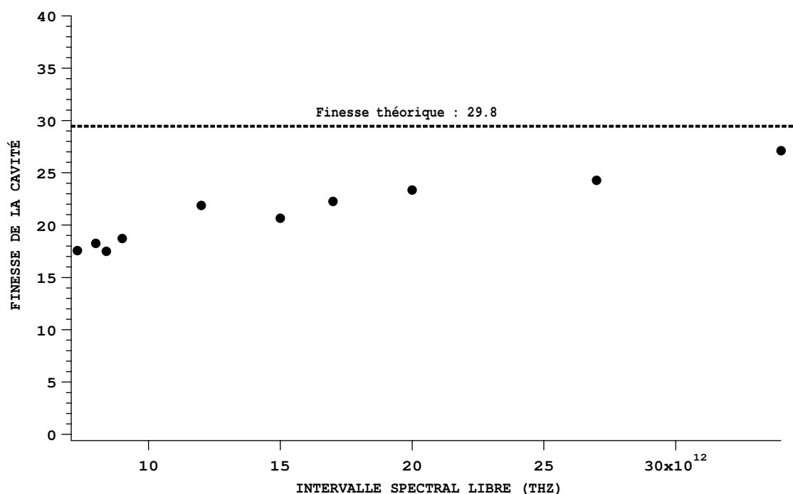
FIG. 5.10 – Evolution de la finesse de la cavité, mesurée à partir des ajustement de la figure 5.9, en fonction de l'intervalle spectral libre ( ISL ). Les valeurs mesurées sont compatibles avec la finesse théorique, qui est de 29.8.
