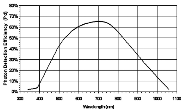
FIG. 3.7 – Efficacité quantique des photodiodes à avalanche AQR14 en fonction de la longueur d'onde (source : Perkin Elmer).
