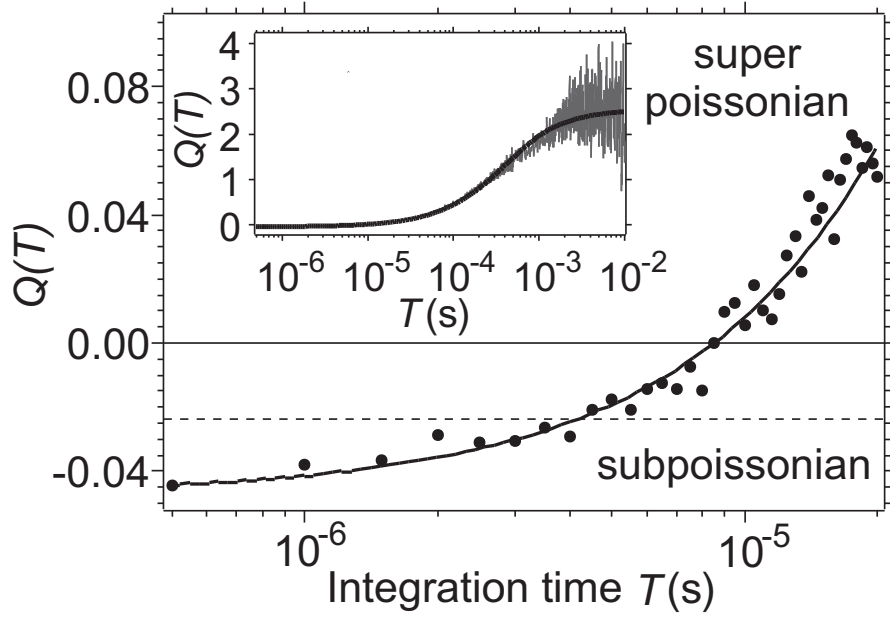
FIG. 4.6 – Paramètre de Mandel de la source moléculaire de photons uniques en fonction de la durée d'intégration T . La courbe est présentée dans son intégralité dans l'insert, tandis que la figure principale correspond à un agrandissement du comportement aux temps courts. La courbe en trait plein représente le résultat de l'ajustement des formules analytiques aux données du modèle ON - OFF. Le trait horizontal pointillé matérialise la limite poissonnienne du facteur de Mandel compte tenu de la saturation introduite par les temps morts des photodétecteurs.
