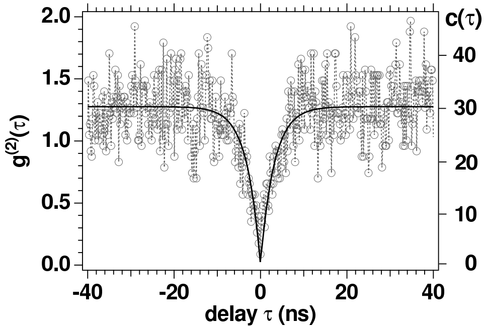
FIG. 3.9 – -o- : fonction d'autocorrélation en intensité g^{(2)}(\tau) obtenue pour une molécule de terrylène dans un film mince de polymère PMMA [71]. Les valeurs de g^{(2)}(\tau) sont déduites du nombre de coïncidences c(\tau) (échelle de droite) enregistrées pendant la durée de l'expérience. Temps d'intégration : 100.4 s. On observe le « dégroupement de photons » correspondant à l'absence de coïncidences au retard \tau = 0 et caractéristique de l'unicité de l'émetteur. Le fait que pour |\tau| \geq 40 ns, la fonction d'autocorrélation g^{(2)}(\tau) prenne une valeur supérieure à l'unité – valeur correspondant à ce que donnerait une source de lumière dont les fluctuations d'intensité suivant une statistique poissonnienne – est dû au passage de la molécule par le niveau triplet métastable. Dès que la molécule quitte ce niveau piège, elle peut de nouveau se mettre à fluorescer. À l'échelle de temps de la durée de vie du niveau triplet, les photons semblent être émis par paquets (« groupement de photons »). En trait plein : ajustement des données expérimentales par un modèle faisant intervenir les trois niveaux S_0 , S_1 et T_1 du diagramme de JABLONSKI.
