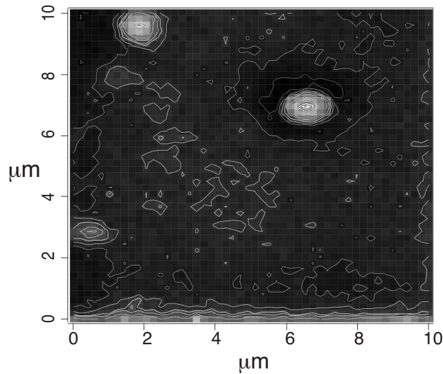
FIG. 5.5 – « Scan » faisant apparaître les variations de niveau de fluorescence lors du balayage par le faisceau laser d'un échantillon de nanocristaux déposés sur un miroir diélectrique. Cette image, a été enregistrée après avoir préalablement « blanchi » le fond de fluorescence du miroir diélectrique et du film polymère entourant les nanocristaux. Elle illustre le fait que seuls les centres colorés NV survivent à cette irradiation, qui permet d'améliorer considérablement le rapport signal à bruit dans la détection des photons émis par le centre coloré.
