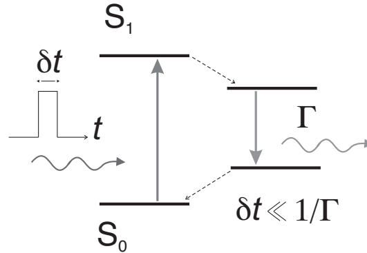
FIG. 3.11 – Schéma de principe d'une source de photons uniques déclenchée, fondée sur la modélisation des niveaux d'énergie d'un fluorophore par un système à quatre niveaux. Une impulsion excitatrice suffisamment brève et intense porte le système dans un état vibrationnel du niveau excité S_1 . De là, il se désexcite d'abord rapidement de façon non-radiative (flèches en pointillés), puis émet un photon unique dans la durée de vie \tau_0 \equiv 1/\Gamma du niveau S_1 avant de revenir dans l'état fondamental du niveau S_0 . Dans la limite où la durée de l'impulsion d'excitation \delta t est très courte devant la durée de vie de fluorescence \tau_0 = 1/\Gamma , le système ne peut émettre qu'un seul photon par impulsion d'excitation.
