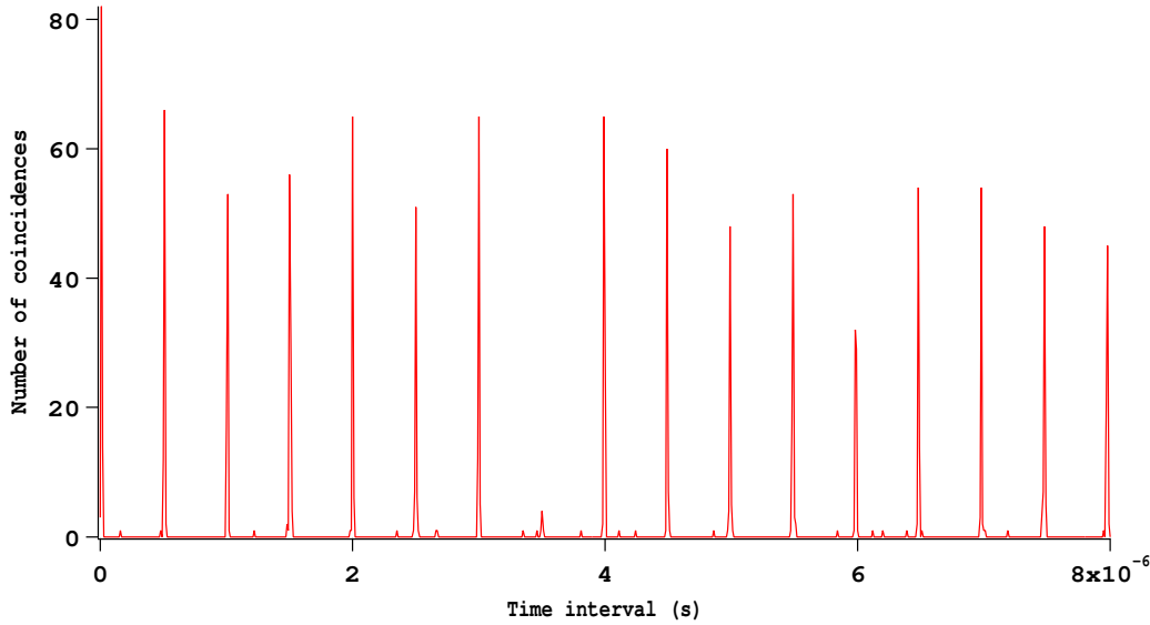
FIG. 4.3 – Histogramme des intervalles de temps séparant deux photodétections, au voisinage du délai nul. Cet histogramme a été calculé numériquement à partir des données \{t_i\} enregistrée par le TIA. La fenêtre temporelle associée a pas de l'histogramme (« timebin ») est de 10 ns.
