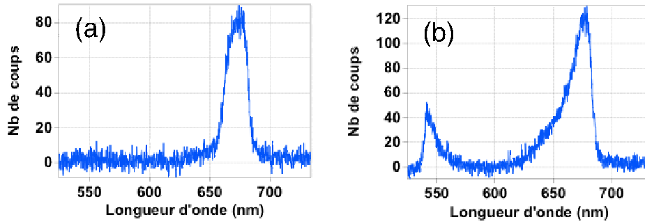
FIG. 5.11 – (a) Spectre en transmission de la microcavité « froide » éclairée en lumière blanche. Ce spectre est obtenu en focalisant dans la cavité un faisceau parallèle de lumière blanche à l'aide d'un autre objectif de microscope de longue distance de travail placé au-dessus du miroir « R_{\max} ». La lumière transmise est collectée par l'objectif principal (distance de travail maximale 3.1 mm, \times 40 , ouverture numérique 0.60) et envoyée vers le spectrographe imageur représenté sur la figure §3.5. Le spectre obtenu a une largeur à mi-hauteur d'environ 20 nm. (b) Spectre de la fluorescence d'un centre NV unique. Le pic autour de 550 nm est un artefact dû au spectrographe (lumière de pompe à 514.5 nm diffusée à l'intérieur du spectrographe) et n'a pas de rapport avec le spectre du centre NV. Ces spectres sont obtenus après une accumulation d'une durée d'intégration de 10 minutes sur la matrice CCD refroidie à -60^\circ\text{C} .
