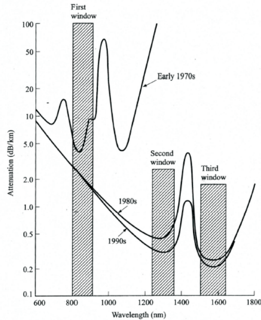
FIG. 8.1 – Transmission des fibres optiques commerciales en fonction de la longueur d'onde. On voit clairement apparaître l'existence de deux « fenêtres » respectivement autour de 1.3 et 1.55 \mu\text{m} .
