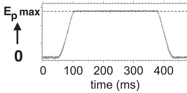
FIG. 3.15 – Rampe d’excitation appliquée pour l’excitation d’une molécule unique. L’acquisition des données est effectuée durant le plateau d’énergie E_p^{\max} = 5.6 pJ. Cette énergie permet d’assurer la saturation de la transition S_0 \rightarrow S_1 de la molécule pour chaque impulsion de pompe appliquée.
