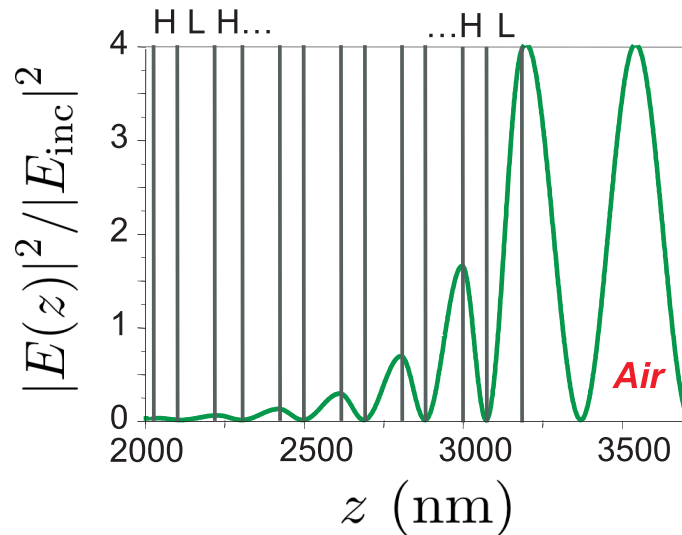
FIG. 5.3 – Structure du miroir de Bragg sur lequel sont déposés les nanocristaux de diamant. Ce miroir est formé d'une alternance d'une couche diélectrique d'indice de réfraction élevé d'oxyde de niobium ( H = \text{Nb}_2\text{O}_5 , n_H = 2.39 ) et d'une couche de silice d'indice de réfraction plus faible ( L = \text{SiO}_2 , n_L = 1.45 ). La courbe en trait plein représente le module au carré du champ électrique en fonction de la position z sur un axe perpendiculaire à la surface du miroir. Cette courbe résulte d'une modélisation de la structure utilisant la technique des matrices de transfert. La réflectivité théorique du miroir ainsi prédite par le modèle est de 99.9996% à 690 nm, le fabricant garantissant une valeur minimale de 99.99%.
