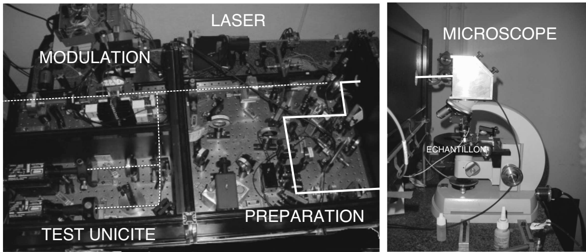
FIG. 7.3 – Photographie du dispositif expérimental utilisé chez Alice.
