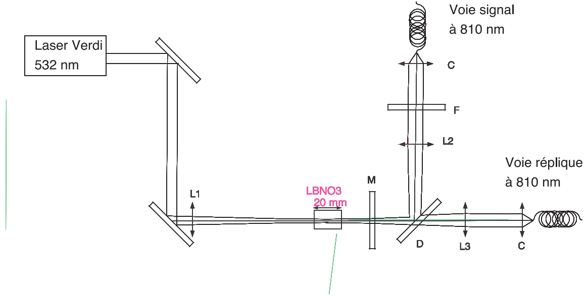
FIG. 8.3 – Montage expérimental : couplage des faisceaux signal (810 nm) et idler (1550 nm) dans des fibres monomodes. L1 : lentille de focale 100 cm, L2 et L3 : lentilles de focale 25 cm. D : miroir dichroïque de coefficient de réflexion 99 % à 810 nm et de transmission 85 % à 1550 nm. M : miroir interférentiel de haute réflectivité à 532 nm, utilisé pour bloquer la lumière de pompe. F : Filtre passe haut. C : coupleur basé sur une lentille asphérique de focale 11 mm. Le waist du faisceau de pompe au niveau du cristal de LiNbO 3 est de 170 \mu m.
