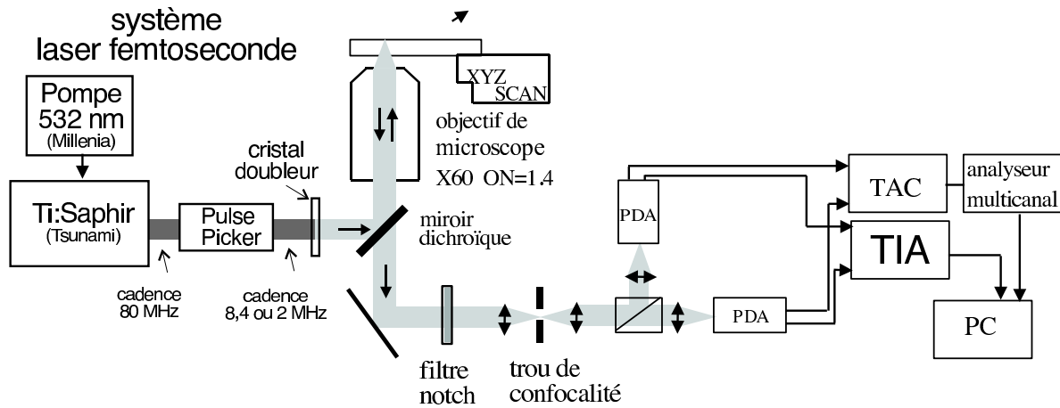
FIG. 3.13 – Schéma de l'expérience en régime d'excitation impulsionnelle. Système d'excitation laser : Ti :Sa : laser impulsionnel saphir dopé titane délivrant des impulsions de durée \approx 150 fs ; PP : sélecteur d'impulsions réduisant la cadence d'excitation de la molécule ; S : cristal doubleur de fréquence \text{LiIO}_3 ; EO : cristal électro-optique suivi d'un polariseur P. Système d'excitation/détection confocal : PZT : platine trois axes piézoélectrique sur laquelle est posée l'échantillon ; Obj. : objectif de microscope à immersion \times 60 , \text{ON}=1.4 ; DM : miroir dichroïque ; PH : trou de confocalité ; NF : filtre réjecteur Notch ; BS : séparateur 50/50 de faisceau insensible à la polarisation ; SPAD : photodiode à avalanche en régime de comptage de photons. TAC : convertisseur temps-amplitude relié à l'analyseur multi-canal MA ; TIA : analyseur d'intervalles temporels (« Time Interval Analyser ») ; PC : ordinateur.
