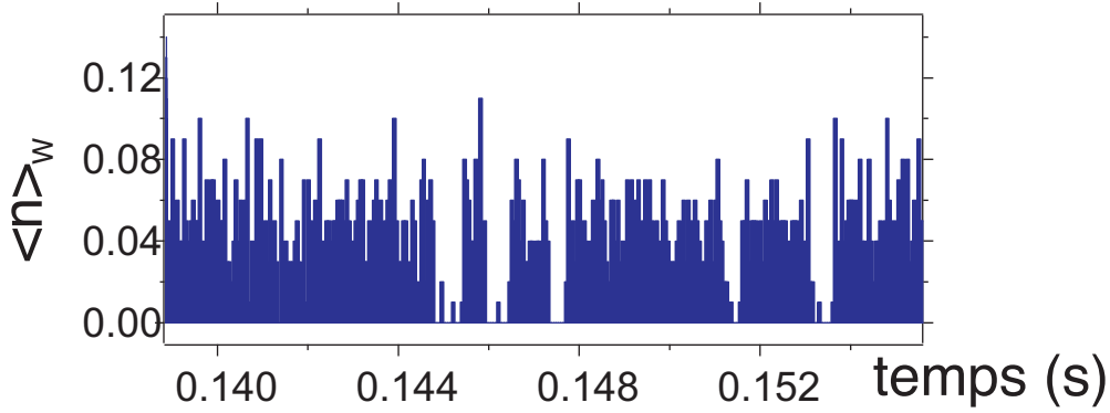
FIG. 4.4 – Périodes « noires » dans l'émission de la source moléculaire de photons uniques. On a représenté le nombre moyen de photons détectés par impulsion, la durée sur laquelle est effectuée la moyenne étant de 100 périodes d'excitation, soit environ 50 \mu\text{s} . À cette échelle de temps, le phénomène d'intermittence dans la fluorescence de la molécule apparaît clairement.
