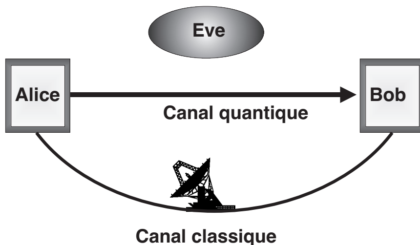
FIG. 2.3 – Cas de figure envisagé en cryptographie quantique : Alice et Bob souhaitent communiquer de façon confidentielle. À cette fin, ils utilisent un canal classique et un canal quantique afin d'établir une clé secrète. Eve, l'espion, tente d'obtenir de l'information sur la clé. Si elle peut écouter librement le canal classique, l'espionnage du canal quantique introduit en revanche des perturbations qu'Alice et Bob peuvent repérer. Alice et Bob vont ainsi pouvoir limiter l'information qu'Eve peut recueillir.
