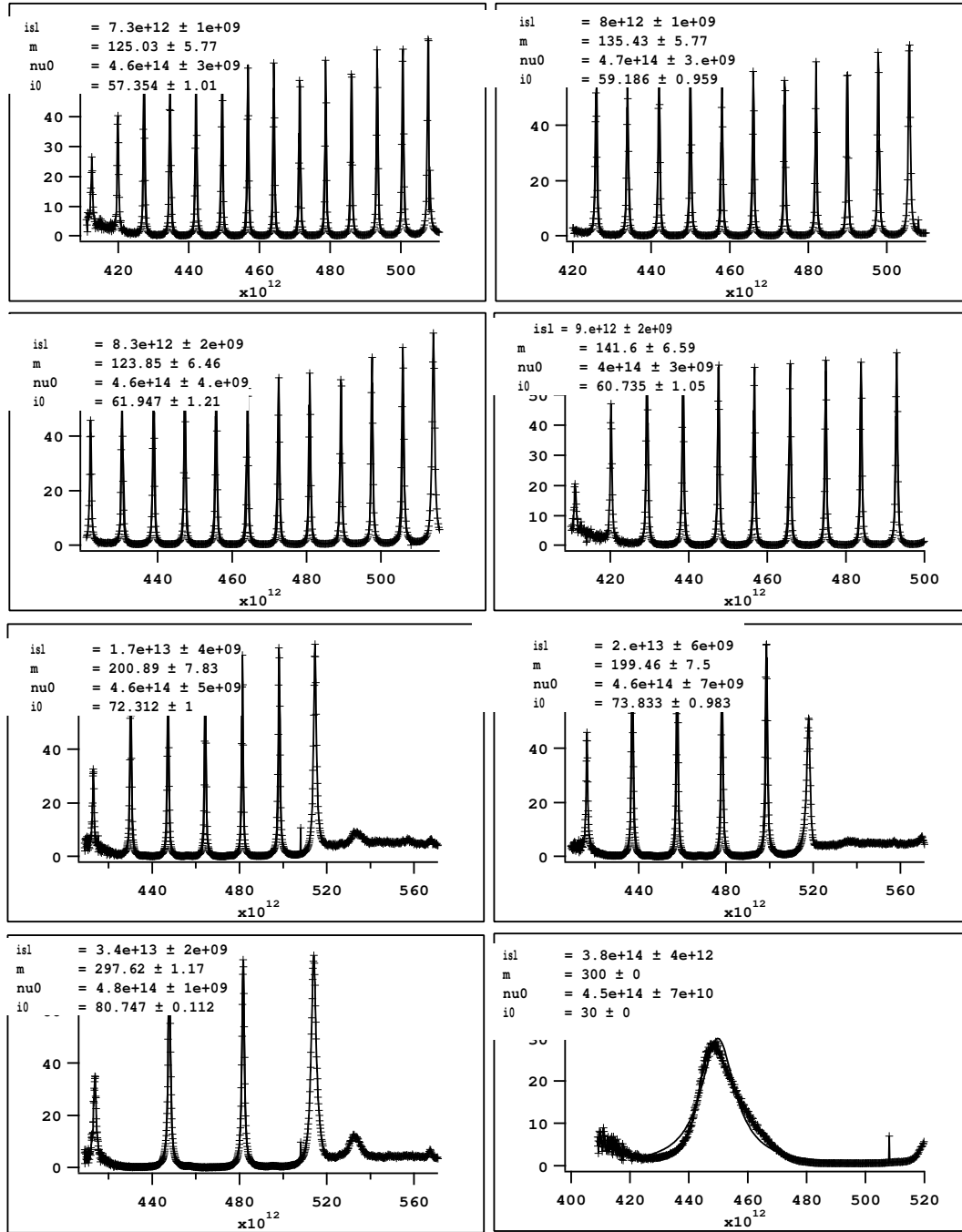
FIG. 5.9 – Spectres de transmission de la cavité planaire, mesurés pour un éclairage normal en lumière blanche. Les différents spectres correspondent à différentes épaisseurs d'air entre les deux miroirs. Chacune de ces courbes est ajustée à partir de l'équation 5.3 et les paramètres de l'ajustement sont portés sur le graphique correspondant. En haut à gauche, le spectre présente de nombreux pics, l'intervalle spectral libre ( ISL ) est faible car les miroirs sont éloignés d'une distance égale à plusieurs multiples de la longueur d'onde. En bas à droite, l'intervalle spectral libre correspond à un réglage proche de la « configuration \lambda/2 ».
