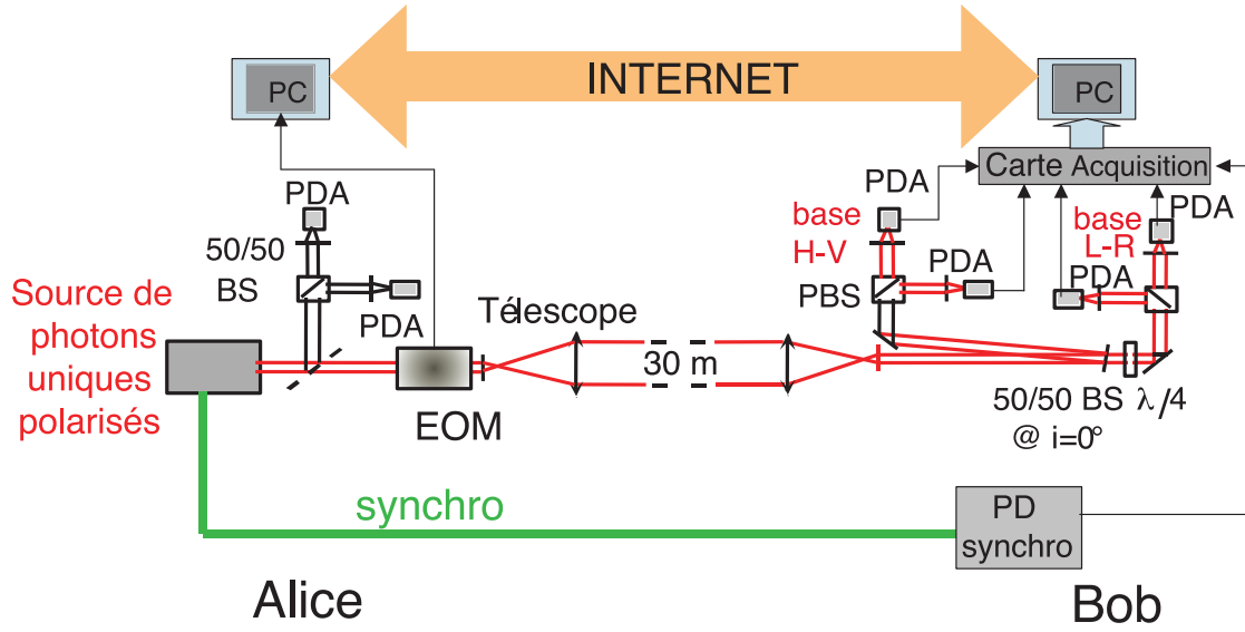
FIG. 7.2 – Schéma du dispositif expérimental permettant la distribution quantique de clés en espace libre entre les deux ailes du bâtiment de l'Institut d'Optique (cf. figure 7.1).
