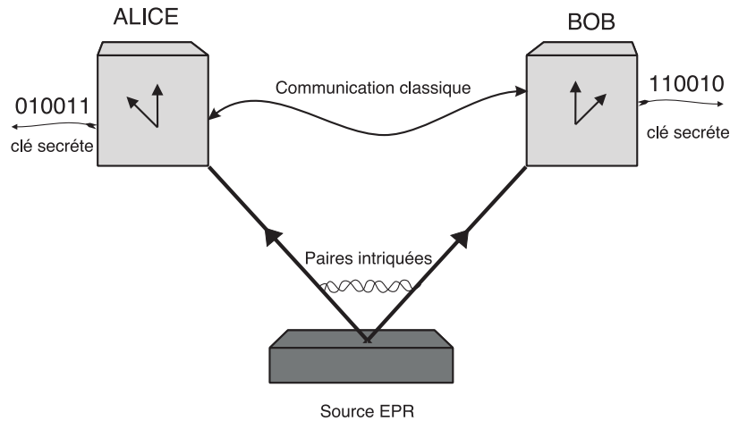
FIG. 6.4 – Représentation schématique d'un système de distribution quantique de clé fondé sur l'usage d'une source de paires de photons intriqués. Alice et Bob mesurent l'arrivée des photons dans l'une des deux bases non orthogonales, comme dans le protocole BB84. Une partie des résultats de mesure permet de vérifier que la source présente bien des corrélations non-locales conduisant à une violation des inégalités de Bell et de s'assurer ainsi de l'absence d'un éventuel espion. Les chaînes des clés brutes obtenues par Alice et par Bob sont utilisées pour obtenir des clés secrètes après les étapes de correction d'erreur et d'amplification de confidentialité.
