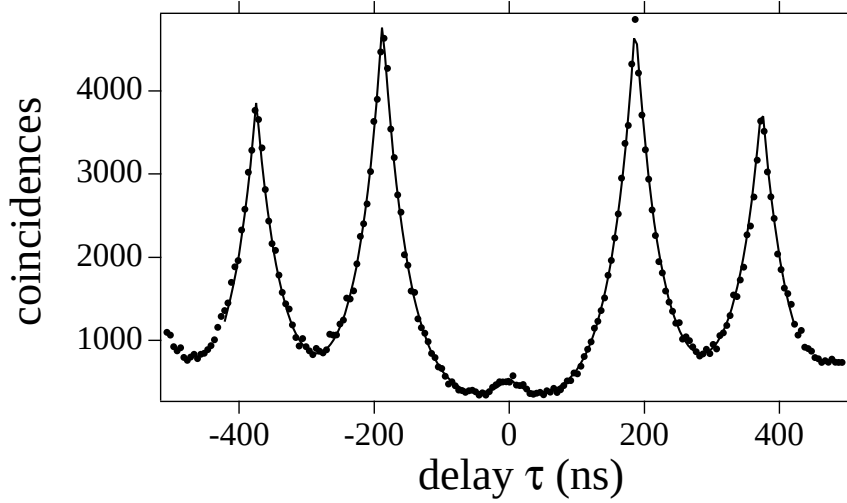
FIG. 7.6 – Histogramme des intervalles de temps entre deux photodétections consécutives enregistrées au niveau d'Alice à l'aide du dispositif de mesure des corrélations d'intensité, de type HANBURY BROWN ET TWISS. Le temps d'intégration est de 175 s. La courbe en trait plein correspond à un ajustement des données expérimentales par un de décroissance exponentiel de chacun des pics, modèle prenant en compte le bruit de fond. Cet ajustement permet d'évaluer à 35 ns la durée de vie radiative du centre coloré NV utilisé. La forte réduction du nombre de coïncidences au voisinage du délai nul est signature du fait que ce centre coloré NV est bien un émetteur individuel qui produit des photons uniques.
