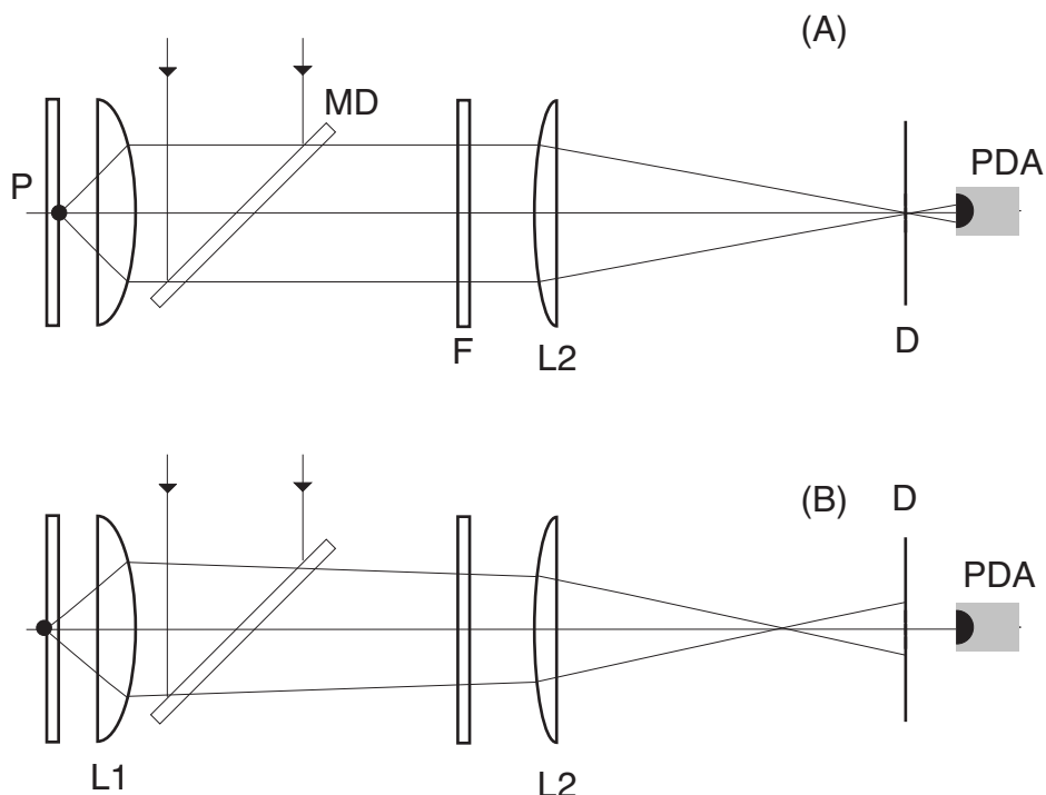
FIG. 3.2 – Schéma expliquant le principe du microscope confocal. (A) La lumière d'excitation est réfléchiée sur un miroir dichroïque vers un objectif de microscope, puis focalisée sur l'échantillon. La lumière rayonnée en retour par l'échantillon (en particulier la lumière de fluorescence) est collectée par le même objectif, filtrée spectralement de la lumière de pompe puis focalisée sur un trou de faible diamètre, qui joue le rôle de filtre spatial. On peut se convaincre, à l'aide du schéma (B) que seuls les rayons lumineux provenant d'une région spatiale limitée autour du plan objet de l'objectif de microscope seront détectés efficacement, ce qui d'isoler la lumière provenant d'un faible volume de l'échantillon[271]. E : échantillon ; L1, L2 : lentilles ; MD : Miroir dichroïque ; F : filtre spectral ; D : diaphragme ; PDA : détecteur (photodiode à avalanche dans notre expérience).
