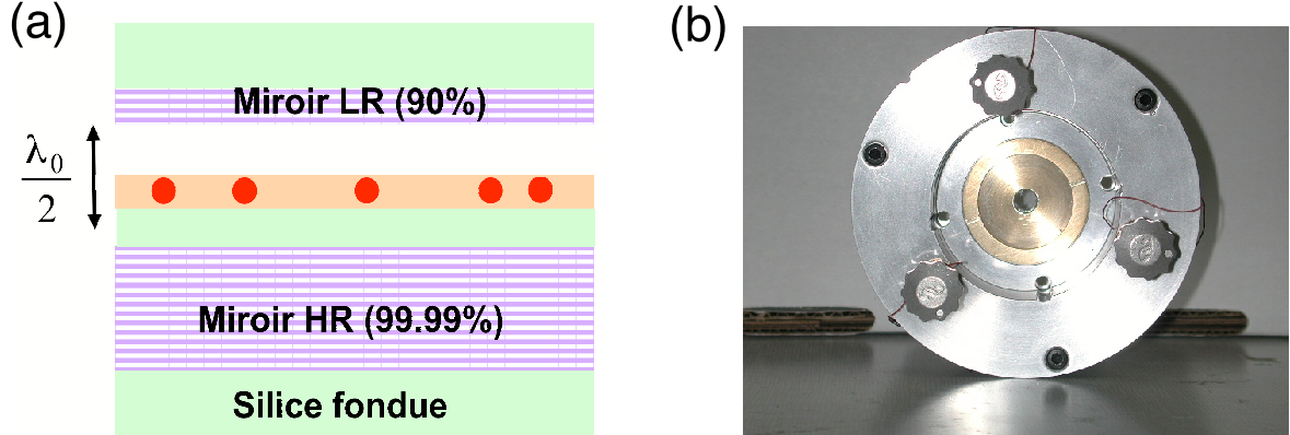
FIG. 5.8 – (a) Configuration testée pour étudier les modifications de la fluorescence de centres colorés, représentés par points gris foncés dans une microcavité dissymétrique plane monomode. Les nanocristaux sont déposés sur le miroir de Bragg de haute-réflexivité (HR) identique à celui utilisé dans la fabrication des échantillons décrite au §5.2. Un miroir de plus faible réflectivité est placé parallèlement au miroir (HR) à environ \lambda_{\text{fluor}}/2 à l'aide de micro- et nano-positionnement. (b) Photographie de la microcavité dont la conception et la fabrication ont été entièrement assurées à l'ENS CACHAN. Les supports de miroirs en laiton, sont amovibles et peuvent être placés sur la partie mobile aussi bien que sur la partie fixe de la cavité. On aperçoit trois vis qui permettent l'ajustement micrométrique ainsi que les fils qui amènent la tension sur les trois cales piézoélectriques permettant d'obtenir un réglage fin de l'épaisseur de la cavité.
