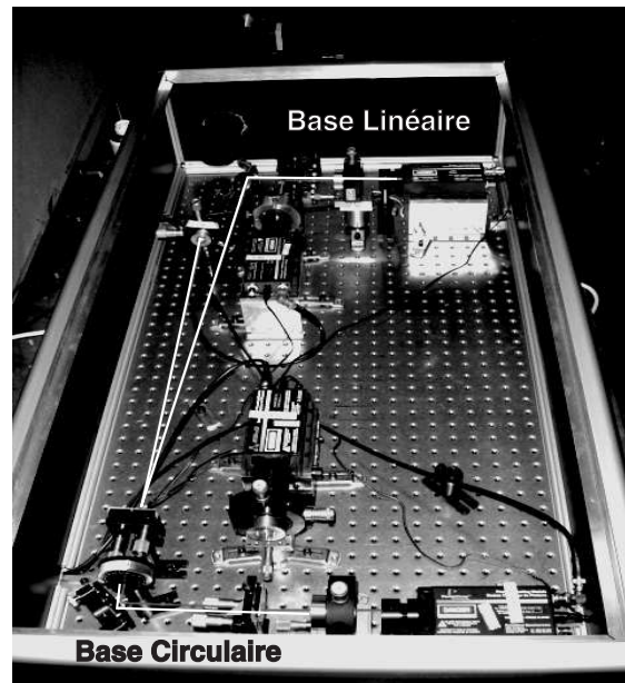
FIG. 7.4 – Photographie du dispositif expérimental utilisé chez Bob.
