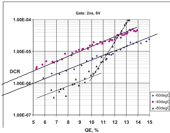
FIG. 8.4 – Performance des photodiodes à avalanche utilisées dans notre expérience : probabilité d’avoir un coup d’obscurité par timeslot, de 2 ns pour différentes valeurs de l’efficacité quantique (Données MAQIQ issues du travail de Darius SUBACIUS)
