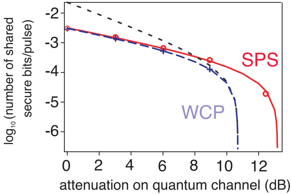
FIG. 7.8 – Taux de clé sûr par impulsion mesuré en bit et présenté sur une échelle logarithmique, en fonction de l'atténuation sur le canal quantique exprimée de décibels. Les courbes sont calculées à partir de l'équation (7.6) et les points sont directement issus des réalisations expérimentales d'échange de clé, en présence d'atténuation sur le canal quantique. La courbe en trait plein et la courbe en tirets larges correspondent respectivement aux performances de la source de photon uniques et d'une source d'impulsions cohérentes atténuées de même taux de comptage. La courbe en tirets courts est obtenue en optimisant G par rapport au paramètre \mu dans l'équation (7.6).
