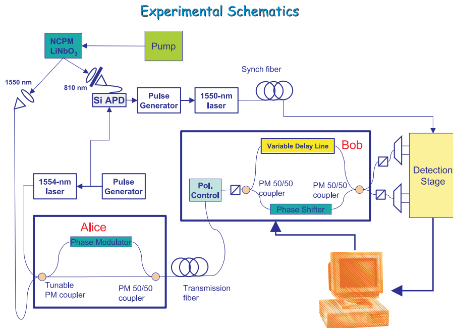
FIG. 8.7 – Dispositif expérimental pour la mesure du taux d'erreur sur une distance de 76 km
