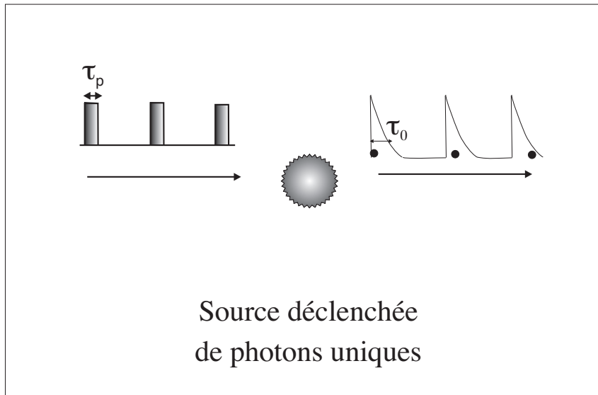
FIG. 1.1 – Schéma de principe d'une source de photons uniques déclenchée : un émetteur unique est porté dans son état excité par une impulsion de pompe, dont la durée \tau_p doit être très brève devant la durée de vie de l'état excité \tau_0 . L'émetteur unique va alors générer, sur une durée typique de l'ordre de \tau_0 , un photon et un seul, dont l'émission a été « déclenchée » par l'impulsion excitatrice.
