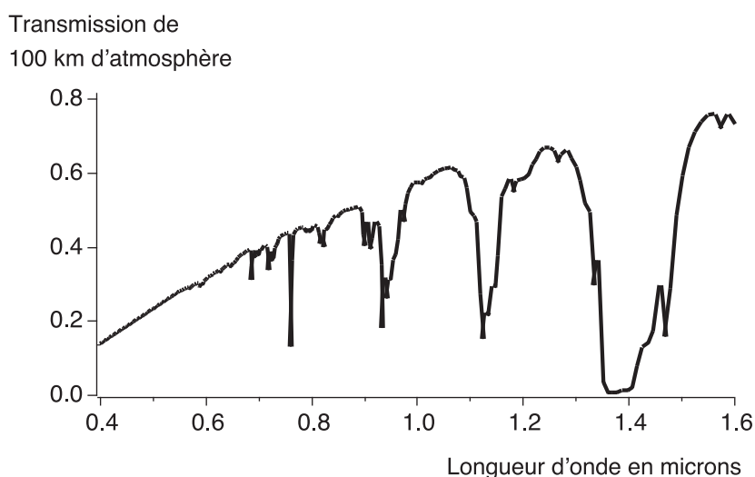
FIG. 6.3 – Transmission de l’atmosphère terrestre sur 100 km (mesurée en pointé vertical), en fonction de la longueur d’onde. On voit apparaître de nettes diminutions dues notamment aux bandes d’absorption de l’eau et des autres composés chimiques présents dans l’atmosphère. Autour de 700 nm, (émission d’un centre coloré NV), l’atténuation est de l’ordre de 4.5 dB pour 100 km.
