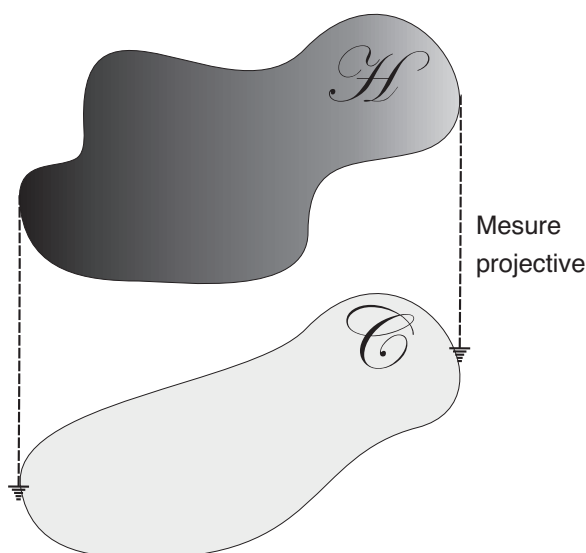
FIG. 6.5 – Représentation schématique de la relation entre le monde quantique, où l'espace des états possibles \mathcal{H} est un espace de Hillbert, et l'espace classique \mathcal{C} qui correspond à l'espace des distributions de probabilités des résultats des mesures, résultats qui sont stockés sous forme classique. La nature projective des mesures effectuées sur les objets quantiques implique que la « taille » de l'espace \mathcal{C} est très inférieure à celle de l'espace \mathcal{H} . Dès lors, seules les preuves dérivées dans l'espace \mathcal{H} peuvent revêtir un caractère de généralité.
