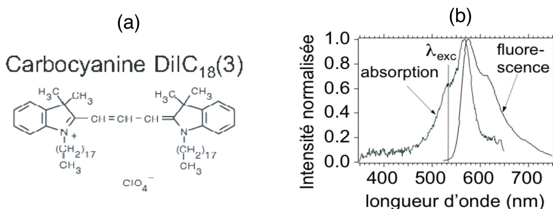
FIG. 3.3 – (a) Structure chimique de la molécule de carbocyanine, de formule DiIC 18 (3). (b) Spectres de fluorescence et d'absorption de cette molécule. Le décalage vers le rouge du spectre de fluorescence par rapport au spectre d'absorption, communément appelé décalage de STOKES , se comprend aisément à partir de la figure 3.1. Ce décalage permet de réaliser une excitation de la molécule à l'aide d'un laser à 532 nm, en dehors de la bande de fluorescence. Ainsi, les photons « parasites » à la longueur d'onde d'excitation, dus essentiellement à la diffusion Rayleigh par l'échantillon, pourront être supprimés de manière sélective au moyen d'un filtre spectral adapté.
