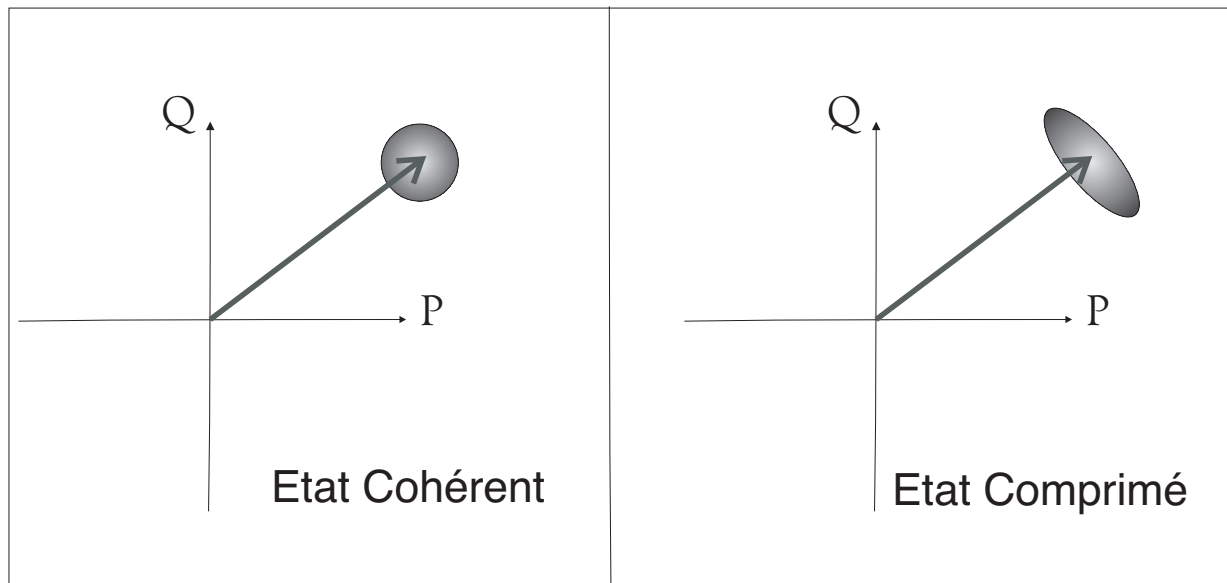
FIG. 2.1 – Représentation, dans l'espace des phases des quadratures P et Q , d'un état cohérent et d'un état comprimé. À gauche, l'état cohérent est un état classique pour lequel les fluctuations \Delta P et \Delta Q sont identiques et correspondent à la « limite quantique standard ». À droite, nous avons représenté un état dit « comprimé en intensité » pour lequel les fluctuations des deux quadratures ne sont pas symétriques. Pour un tel état, l'incertitude de mesure due au bruit quantique sur l'intensité du champ est inférieure à la limite du bruit de photons, tandis que l'incertitude se reporte en quelque sorte sur la phase relative des deux quadratures.
