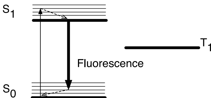
FIG. 3.1 – Diagramme de JABLONSKI des niveaux d'énergie d'une molécule de colorant. Les niveaux S_0 et S_1 correspondent à des états singulet de spin, tandis que le niveau T_1 est associé à une structure triplet. Nous avons représenté en traits plus fins les états vibrationnels excités de S_0 et S_1 . La fluorescence provient de la transition de l'état vibrationnel de plus basse énergie du niveau excité S_1 , vers un état quelconque du niveau fondamental S_0 . Les flèches en tirets représentent des désexcitations non radiatives. Enfin, la transition T_1 \rightarrow S_0 , qui correspond à une transition interdite pour l'opérateur dipolaire électrique donne lieu au phénomène de phosphorescence .
