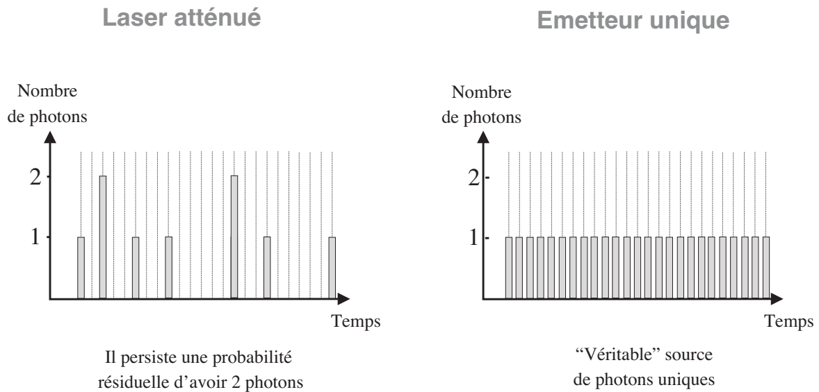
FIG. 2.4 – Différence entre une source poissonnienne atténuée et une vraie source de photons uniques. Dans le cas d’une source atténuée, on doit prendre \langle n \rangle \ll 1 pour limiter le nombre d’impulsions contenant deux photons, qui restent néanmoins présentes de manière résiduelle. Dans le même temps, l’atténuation diminue la quantité d’impulsions « remplies » et par là même le débit des communications réalisables. A l’inverse, une source de photons uniques déclenchée idéale ne souffre pas de ces deux défauts : pour chaque impulsion d’excitation, elle conduit à l’émission d’un photon et un seul.
