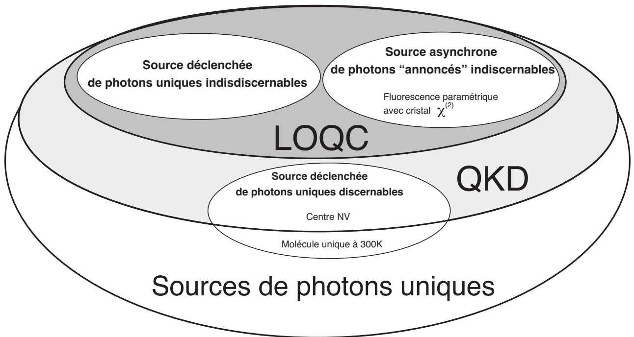
FIG. 2.7 – Classification des sources de photons uniques en fonction des applications pour lesquelles elles sont adaptées. Nous avons placé sur ce schéma les trois systèmes expérimentaux sur lesquels nous avons travaillé dans le cadre de cette thèse : molécule fluorescente unique, centre coloré unique du diamant et source de photons annoncés basée sur la fluorescence paramétrique dans un cristal non-linéaire.
