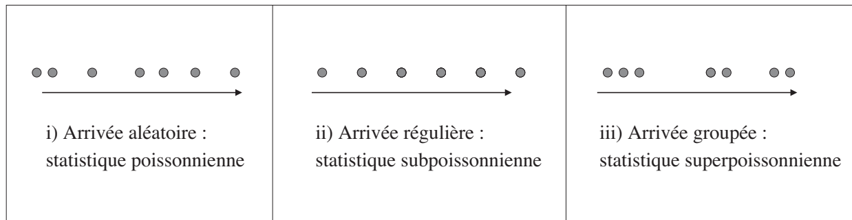
FIG. 2.2 – Représentation corpusculaire du flux de photons dans un faisceau lumineux, distinguant trois cas de figures : i) Source « classique » de lumière, conduisant à une statistique de Poisson des photons émis, tous les instants d’émission étant équiprobables. ii) Émission régulière de photons, correspondant à des fluctuations d’intensité sub-poissonniennes. iii) Groupement de photons, caractéristique par exemple d’une lumière chaotique ou thermique ; les fluctuations d’intensité sont alors supérieures à celles de la référence poissonnienne.
