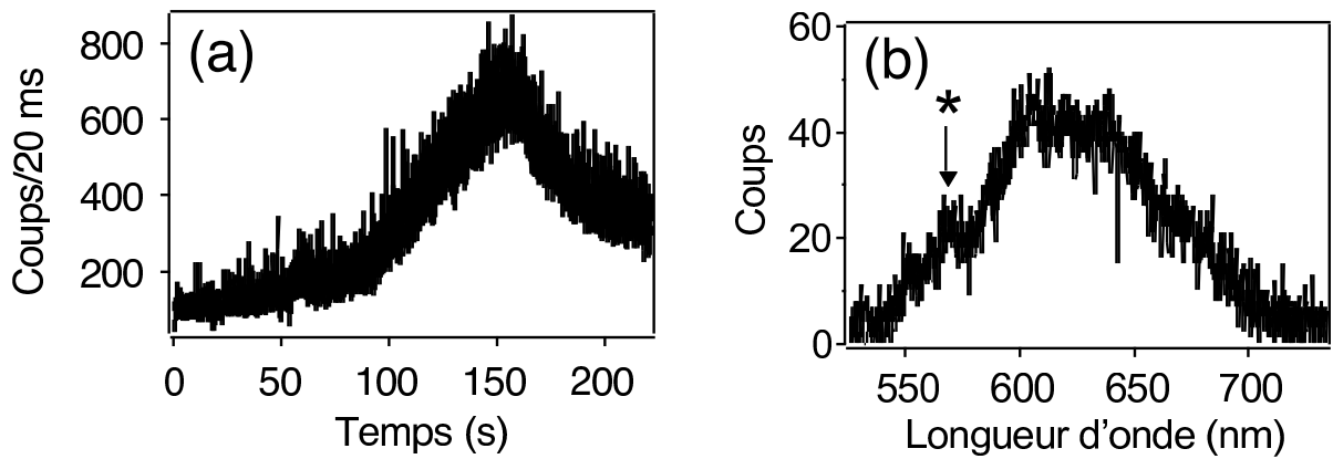
FIG. 5.12 – (a) Variation de l'intensité de la fluorescence collectée en fonction du temps, sous illumination laser femtoseconde focalisée sur l'échantillon. Longueur d'onde 500 nm, énergie par impulsion \approx 55 pJ, fréquence de répétition 8.2 MHz. L'intensité lumineuse au foyer de l'objectif de microscope utilisé pour la focalisation du faisceau d'excitation sur l'échantillon est de l'ordre de 20 \text{ GW} / \text{cm}^2 . Le bruit associé à cette acquisition est en grande partie imputable au phénomène d'intermittence. (b) Spectre de la fluorescence enregistré par le spectrographe imageur, pendant l'éclairage du nanocristal par le faisceau laser femtoseconde et pour une durée d'intégration de 20 minutes. Le spectre a subi un décalage vers le bleu par rapport à celui du centre NV et il est apparu une raie (marquée de l'étoile) autour de 570 nm, caractéristique de la raie zéro-phonon du centre NV^0 neutre.
