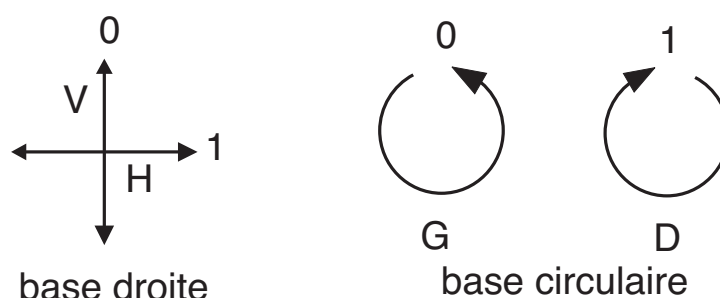
FIG. 6.1 – Bases de polarisation rectilignes et circulaires et bits codés. Ce choix de base, sera utilisé dans l'expérience de cryptographie quantique décrite dans le chapitre suivant pour la réalisation du protocole BB84.
