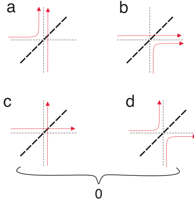
FIG. 2.5 – Deux photons indiscernables, particules bosoniques, semblent se « regrouper » en sortie d’une lame séparatrice. Dans le cas où la lame séparatrice est une lame pour laquelle les coefficients de réflexion et de transmission sont égaux à 50 %, les amplitudes de probabilité correspondant aux termes c et d, pour lesquels les deux photons sont soit transmis soit réfléchis, sont de signes opposés. Ils s’annihilent en interférant destructivement. On observe donc expérimentalement que les photons sortent du même côté de la lame séparatrice (termes a et b).
