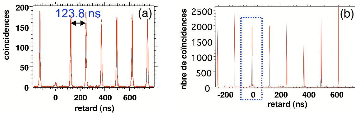
FIG. 3.14 – (a) Histogramme des retards entre photons consécutivement détectés sur l'une puis l'autre photodiode. La lumière provient d'une molécule unique excitée à la cadence de 8 MHz, à la longueur d'onde \lambda = 514 nm, et dans le régime des faibles énergies par impulsion d'excitation. Dans ce régime d'excitation impulsionnelle, la très petite aire du pic au retard nul traduit le dégroupement de photons caractéristique de la lumière provenant d'un seul émetteur quantique. (b) Cas où la lumière provient d'une source classique atténuée. Il s'agit en l'occurrence, d'une fraction du faisceau de pompage réfléchi sur l'échantillon, et ayant été au préalable légèrement décalé en longueur d'onde de la valeur centrale du filtre réjectif « notch » utilisé dans le système de microscopie confocale.
