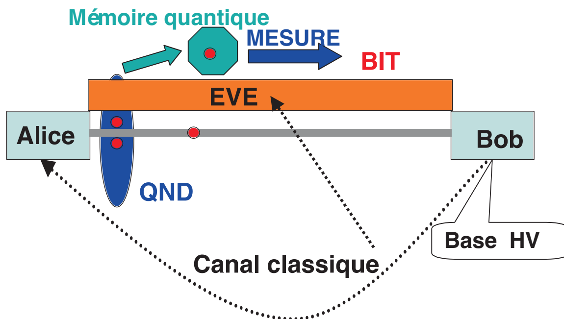
FIG. 6.7 – Principe de l’attaque PNS. Eve réalise une mesure quantique non-destructive (QND) du nombre de photon. Si l’impulsion contient plus d’un photon, Eve en conserve un dans une mémoire quantique et transmet l’autre photon à Bob. Eve attend ensuite que Bob annonce sa base de mesure pour faire la mesure a posteriori, dans la même base. De cette façon, Eve peut acquérir, sans introduire aucune erreur, la totalité de l’information contenue sur les impulsions à deux photons. Une telle attaque suppose qu’Eve est capable de réaliser une mesure QND du nombre de photons et qu’elle dispose d’une mémoire quantique. Une telle hypothèse est en pratique très hardie, mais elle est autorisée par la physique quantique [124, 144].
