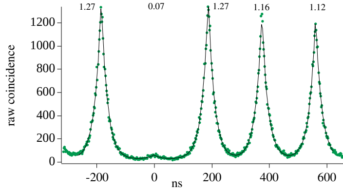
FIG. 5.6 – Fonction d'autocorrélation d'un centre NV unique
