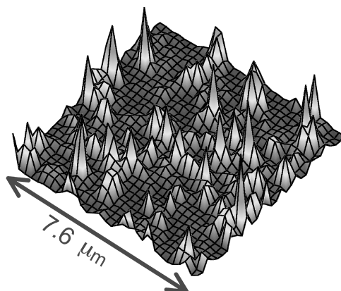
FIG. 3.6 – Pics de fluorescence tels qu'ils apparaissent lors du scan d'un échantillon à l'aide du dispositif de microscopie confocale.
