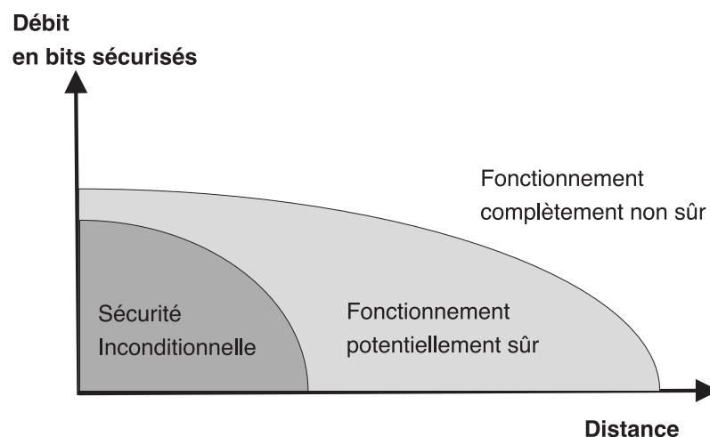
FIG. 6.6 – Les différents régimes de sécurité pour le fonctionnement d'un système réel de distribution quantique de clé. Nous avons choisi la distance entre Alice et Bob comme paramètre de sécurité, avec l'hypothèse implicite que les autres paramètres comme le taux d'erreur ou le nombre moyen de photons par impulsions peuvent être optimisés pour une distance donnée afin de permettre le débit maximal de bits sûrs. Le régime de sécurité inconditionnelle permet de garantir la sécurité des clés indépendamment de toute stratégie d'attaque adoptée par un espion. Le régime de sécurité potentielle correspond au régime pour lequel il n'a pas été exhibé d'attaque suffisamment puissante pour empêcher le partage de clés secrètes. Pour le régime de fonctionnement « complètement non sûr », il existe des attaques rendant impossible l'établissement d'une clé secrète.
