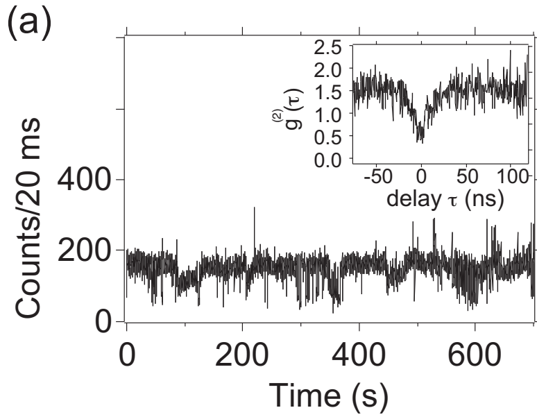
FIG. 5.13 – Enregistrement simultané, en régime d'excitation continue, de l'intensité du signal de fluorescence et de la fonction d'autocorrélation en intensité. Cette acquisition a été effectuée immédiatement après l'illumination d'un centre unique à l'aide du laser femtoseconde . Il apparaît clairement que l'intensité de fluorescence est stable dans ce régime d'excitation. En revanche le « creux » de l'ordre de 0.5 dans la courbe de dégroupement indique que l'on est en présence d'un nanocristal contenant deux centres émetteurs, et donc qu'il y a eu création d'un centre durant l'illumination par le laser femtoseconde ?
