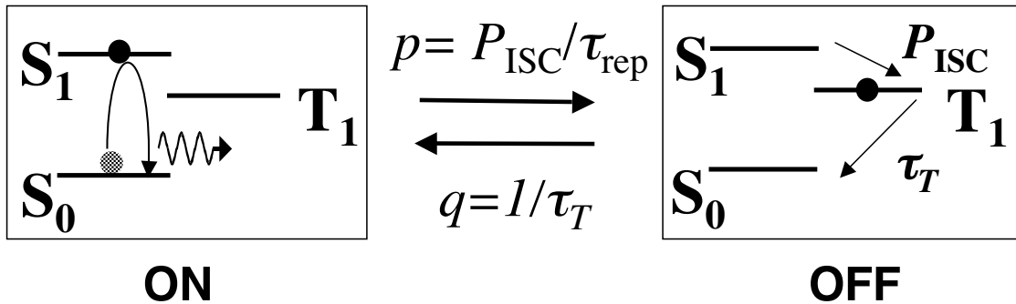
FIG. 4.5 – Structure à trois niveaux utilisée pour modéliser l'intermittence ON - OFF de la molécule. Dans l'état ON, la molécule effectue des cycles d'excitation-émission entre l'état fondamental S_0 et l'état excité S_1 . Dans l'état OFF, la molécule est piégée dans l'état « noir » métastable T_1 . Les transitions de S_1 vers T_1 ont lieu avec une probabilité P_{\text{ISC}} après chaque excitation et correspondent à un taux de transition ON \rightarrow OFF p = P_{\text{ISC}}/\tau_{\text{rep}} . Les transitions inverses, OFF \rightarrow ON, ont lieu à un taux q = 1/\tau_T , où \tau_T est la durée de vie de l'état triplet T_1 .
