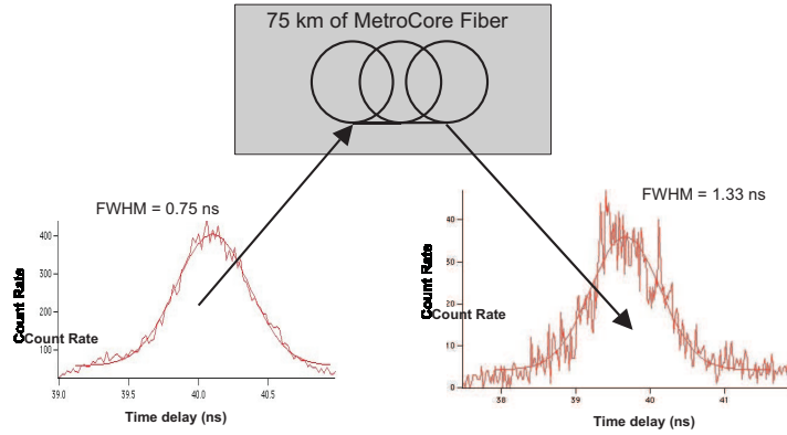
FIG. 8.5 – Enveloppe temporelle des photons sur le canal quantique avant et après propagations dans 76 km de fibre optique. L’enveloppe temporelle des coïncidences 810 nm / 1550 nm est mesurée en variant le retard électronique relatif entre les deux voies. Sur la figure de droite, l’enveloppe temporelle est mesurée directement en sortie de la source de photons annoncés. Sa largeur est limitée par la gigue de 700 ps de la photodiode au silicium placée sur la voie à 810 nm. La figure de gauche est mesurée après 76 km de propagation dans une fibre monomode SMF -28. L’élargissement temporel mesuré est en très bon accord avec la dispersion causée par la fibre, typiquement de 17 ps/nm/km.
