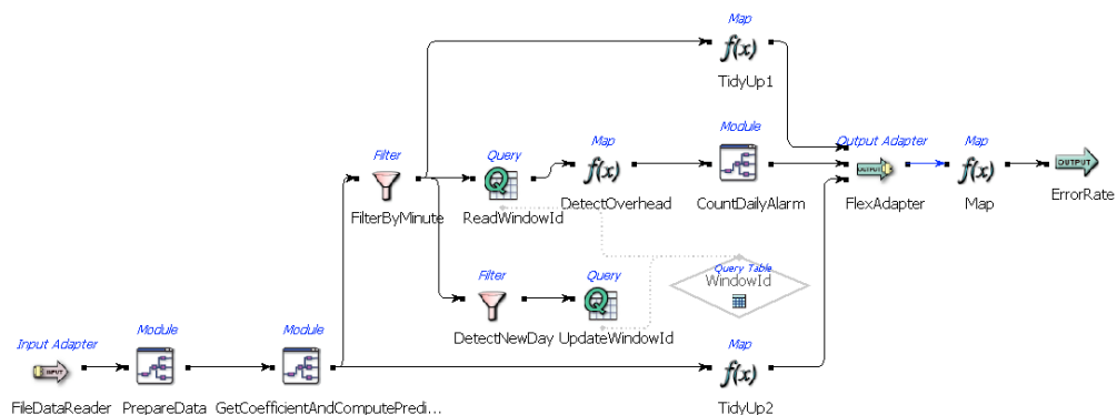
FIG. 5 – Diagramme de l'application de visualisation de la charge d'un centre d'appels.
