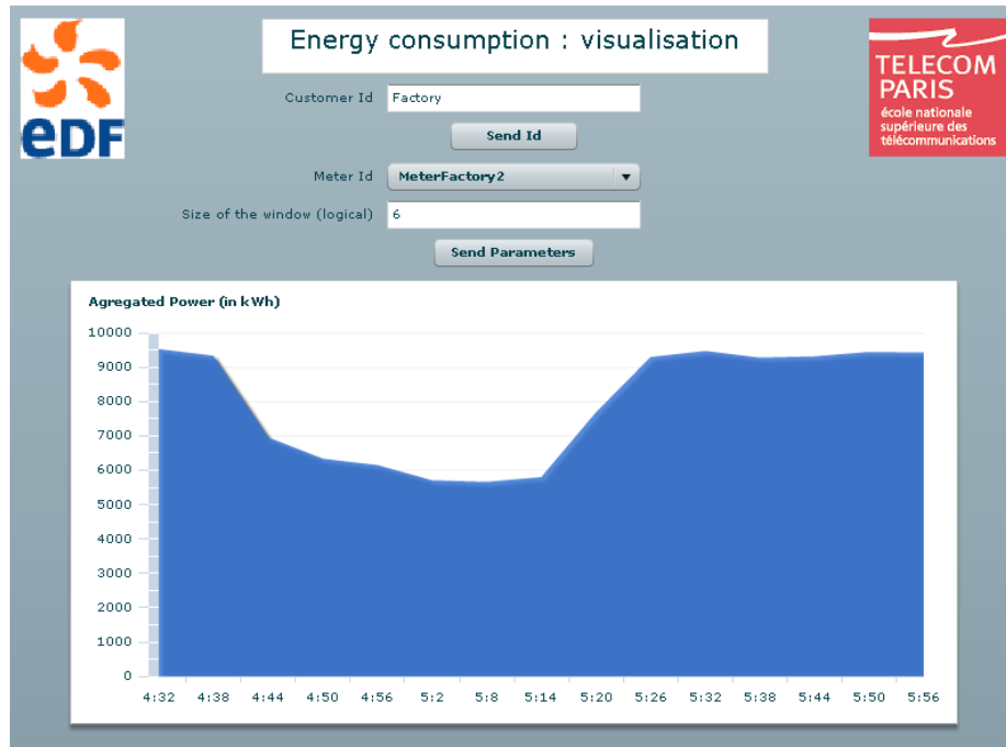
FIG. 4 – Application web de visualisation de consommation. Le client remplit le champ d'identification et clique sur Envoi. La liste de ses compteurs est alimentée. Il sélectionne le compteur dont il souhaite visualiser les mesures et spécifie la taille logique de la fenêtre pour agrégation. Il clique sur Envoi et la visualisation suit son cours.
