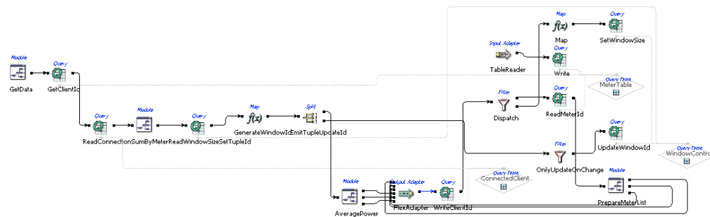
FIG. 3 – Diagramme de l'application de visualisation de consommation.
