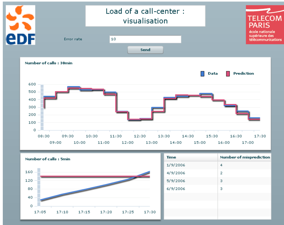
FIG. 6 – Application web de visualisation de la charge d'un centre d'appels. Le graphique principal montre la courbe du nombre d'appels et la courbe du nombre d'appels estimé à raison d'une donnée toutes les demi-heures. Le second graphique montre le nombre d'appels cumulé depuis le début de la demi-heure, toutes les 5 minutes. Le tableau affiche le nombre de fois sur une journée où l'écart relatif entre la réalité et la prédiction dépasse un certain pourcentage. Le pourcentage est un paramètre spécifié par l'utilisateur dans le champ prévu à cet effet et transmis en cliquant sur Envoi.
