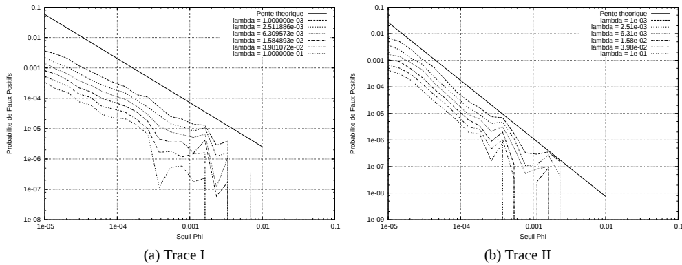
FIG. 2: Probabilité de Faux Positifs en fonction du seuil \phi pour différentes valeurs du taux d'échantillonnage \lambda . Pour chacune des traces, nous avons également tracé une droite de pente -(\beta + \frac{1}{2}) , le paramètre \beta ayant été calculé pour chaque trace de la façon indiquée au § 4.2.
