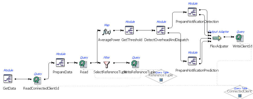
FIG. 1 – Diagramme de l'application de suivi de consommation.
