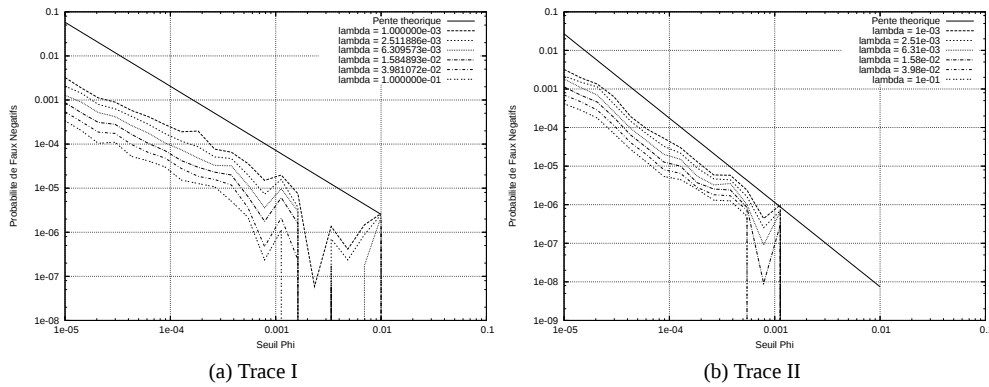
FIG. 3: Probabilité de Faux Négatifs en fonction du seuil \phi pour différentes valeurs du taux d'échantillonnage \lambda . Pour chacune des traces, nous avons également tracé une droite de pente -(\beta + \frac{1}{2}) , le paramètre \beta ayant été calculé pour chaque trace de la façon indiquée au § 4.2.
